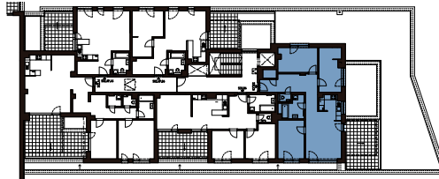
PÔDORYS PODLAŽIA
