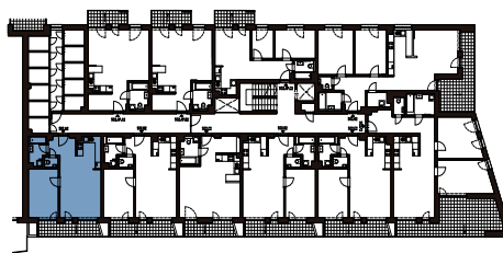
PÔDORYS PODLAŽIA
